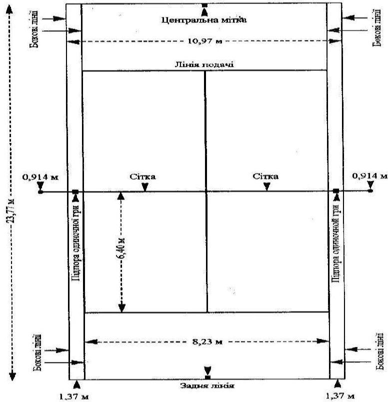
Мал. 1. Схема та розміри тенісного корту
